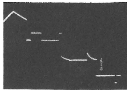
(a) Ces trois oscillogrammes ont été pris en appliquant à chaque fois les quatre mêmes signaux sur les entrées du commutateur, mais en changeant la fréquence de découpage. (a) correspond à ce qu'on doit normalement observer, tandis que sur (b) et (c), on avait choisi une fréquence trop faible et multiple de celle de la base de temps.
